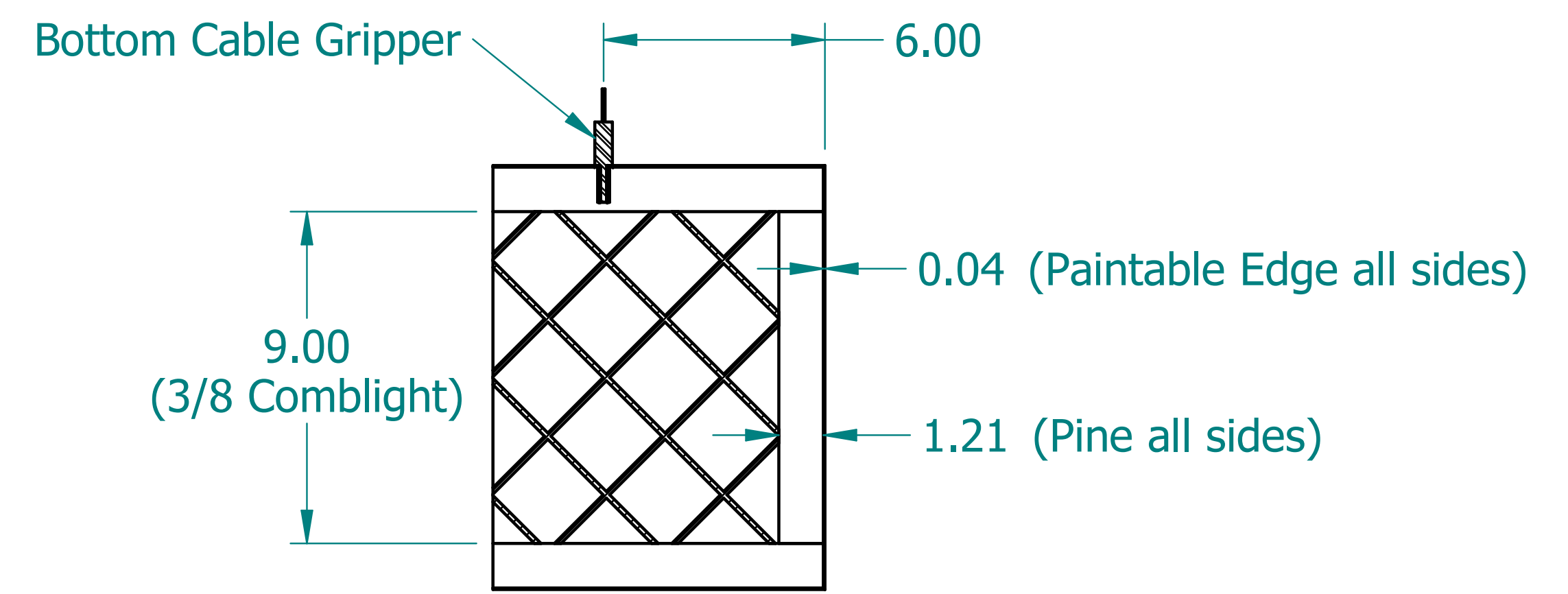
SECTION A-A
