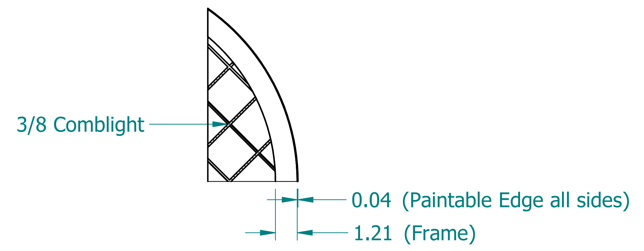
SECTION A-A
