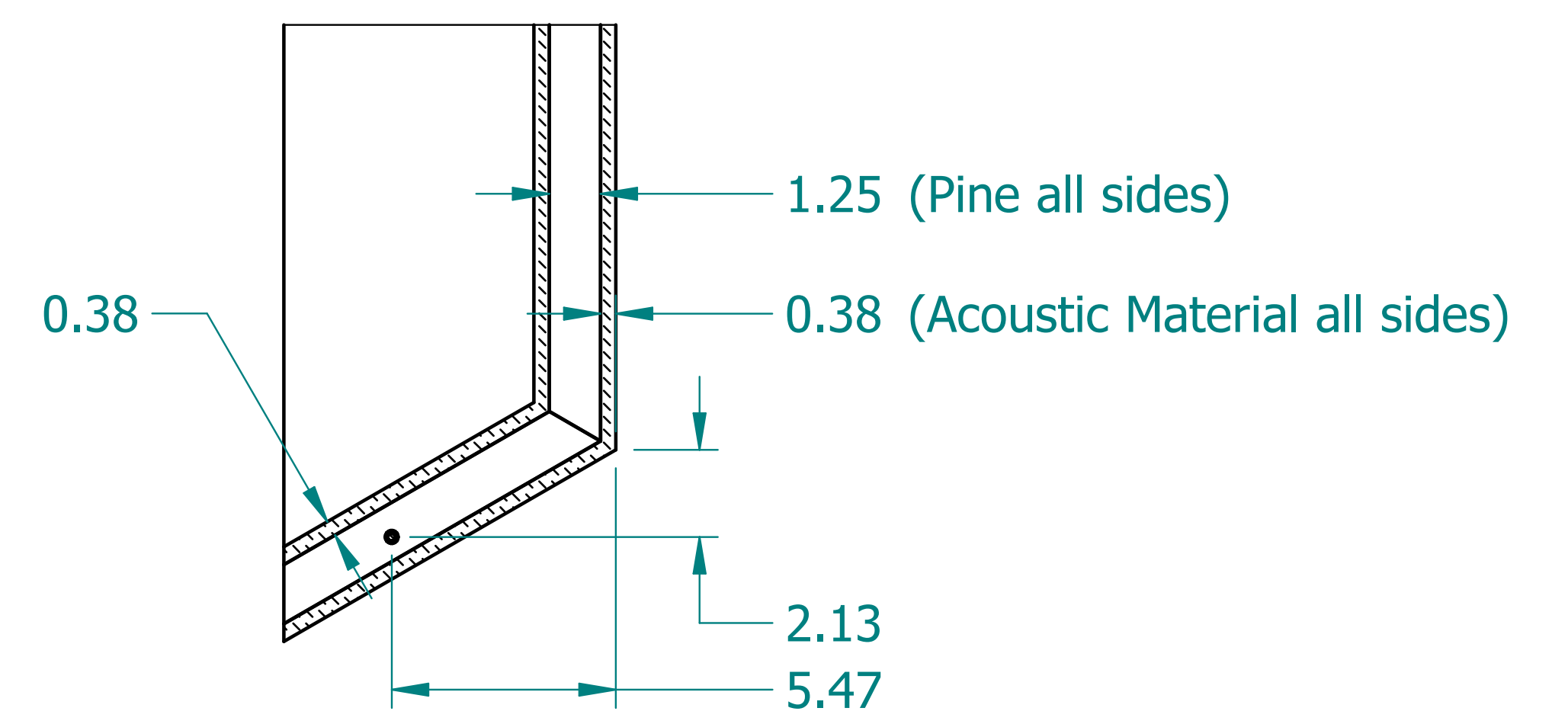
SECTION A-A
